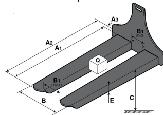
FR: Wrapover forks
